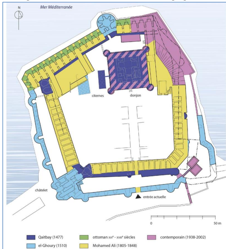
Fig.1 : Le fort Qaitbay
