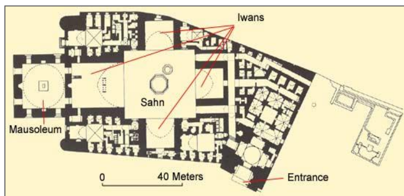
Fig.2 : le plan du complexe Sultan Hassen
