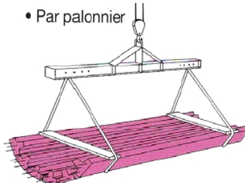
Figure 10 : Mise en œuvre des planchers avec poutrelles préfabriquées 3
