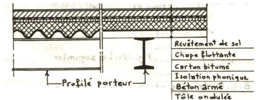
Plancher en tôle ondulée
