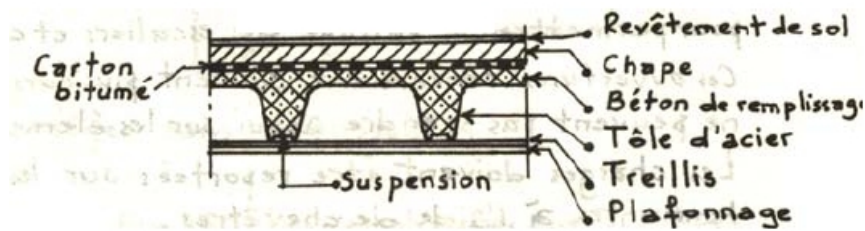
Plancher en tôle pliée
