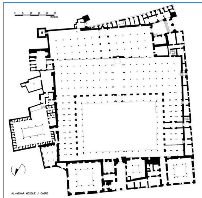
Figure 3 : Plan après les remaniements (mamlouk et ottomane)
