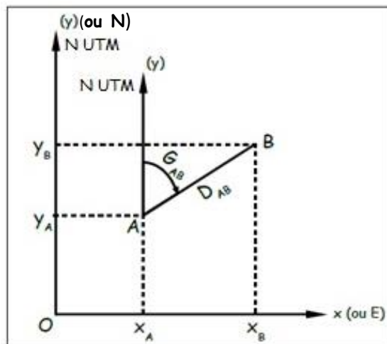
Figure 3.9: Transformation polaire en rectangulaire
