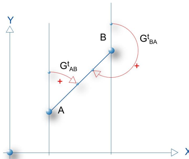
Figure 3.4: Gisement d'une direction
