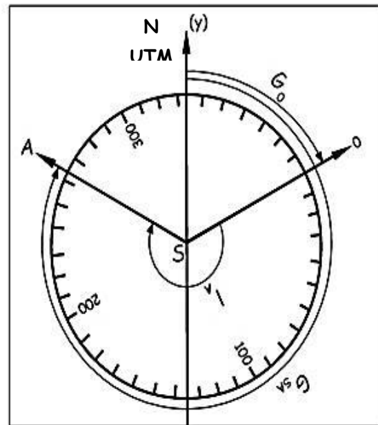
Figure 3.7: Gisement d'origine G_0
