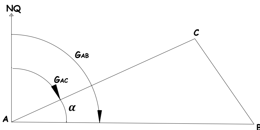
Figure 3.15: différence de deux gisements ou lectures
