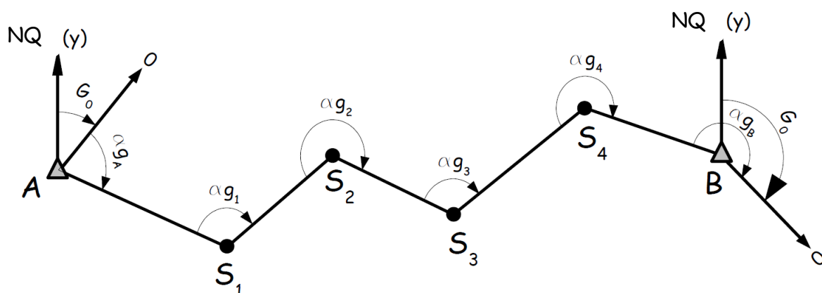
Figure 3.12: Schéma d'un cheminement
