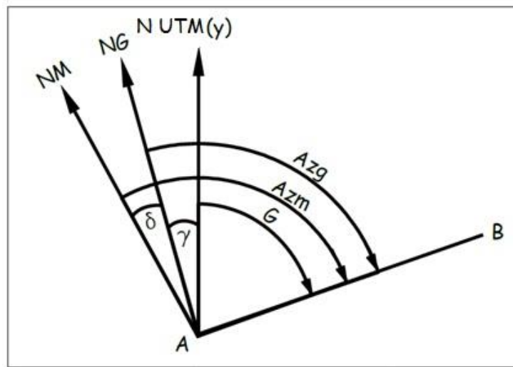
Figure 3.8: ORIENTATION D'UNE DIRECTION
