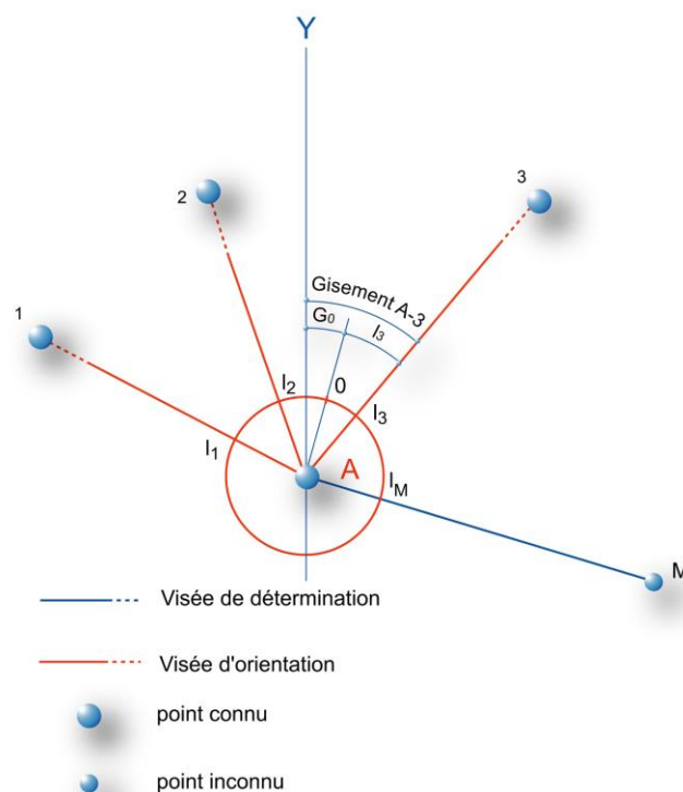
Figure 3.11: G_0 et Rayonnement
