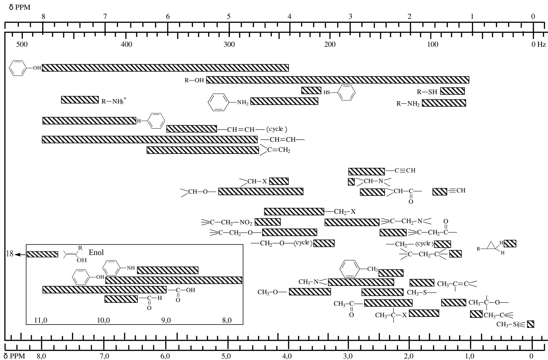
Déplacements chimiques des principaux types de protons en chimie organique (d'après un document Bruker Biospin)
