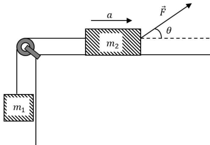
FIGURE 3.13 – Un bloc m_1 en M. R. U. sur une surface horizontale rugueuse et m_2 suspendu dans l'air
