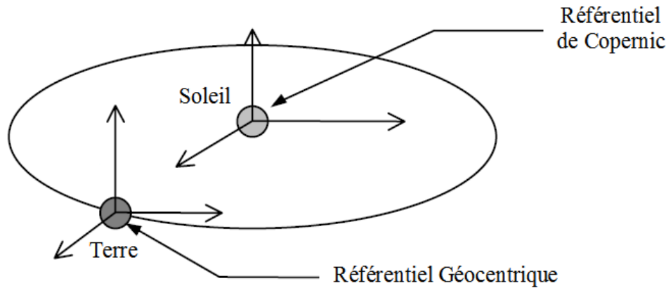
FIGURE 3.1 – Référentiels galiléens
