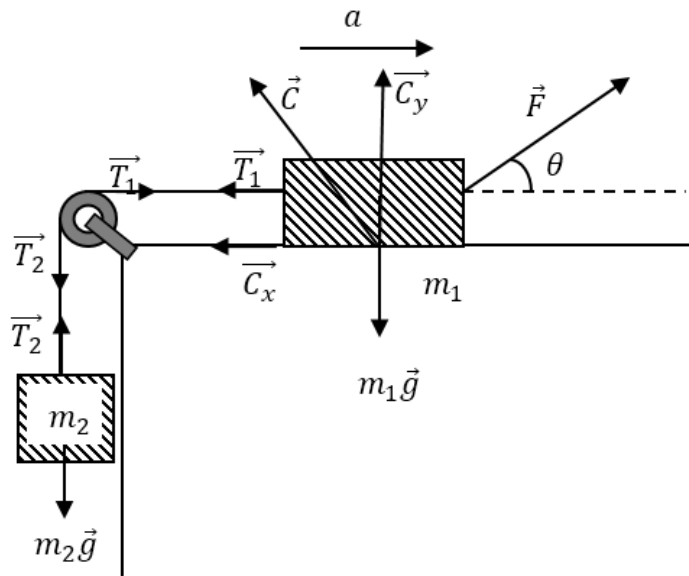
FIGURE 3.14 – Un bloc m_1 en M. R. U. sur une surface horizontale rugueuse et m_2 suspendu dans l'air
