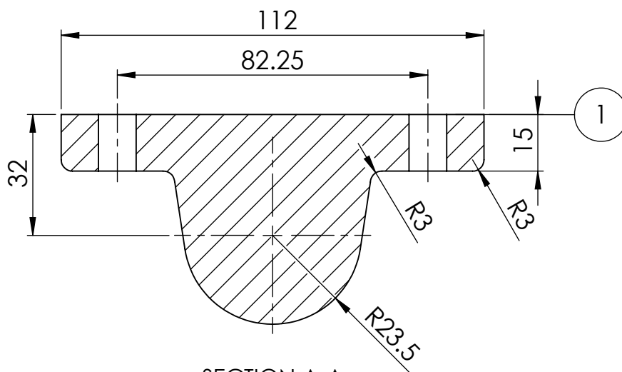
SECTION A-A SCALE 7 : 10
