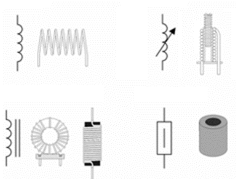
FIGURE 2.5 – Symboles et formes des bobines.
