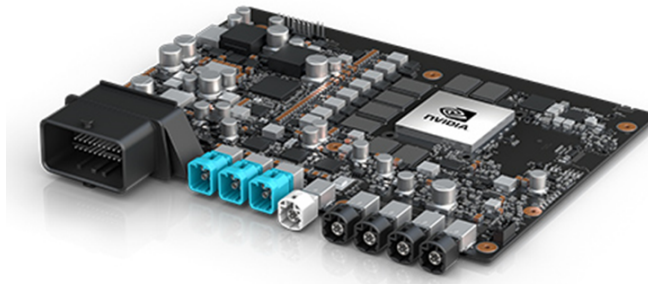
FIGURE 2.15 – Exemple de carte IA automobile : NVIDIA DGX spécialisée dans l’entraînement et l’optimisation des réseaux de neurones. Cette carte équipe la majorité des véhicules avec une autonomie de niveau 3, 4 et 5.
