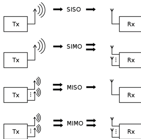
FIGURE 5.1 – Systèmes monovariables et multivariables.
