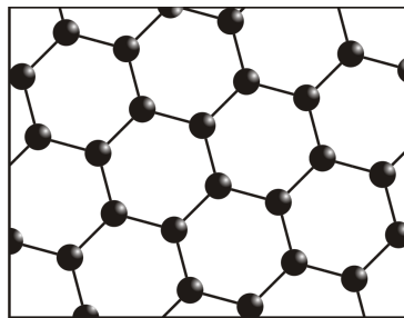
FIGURE 2.12 – Molécule de graphène
