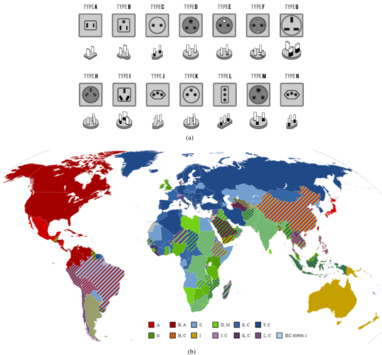
FIGURE 4.4 – (a) Types de prises domestiques et (b) type de prises par pays.
