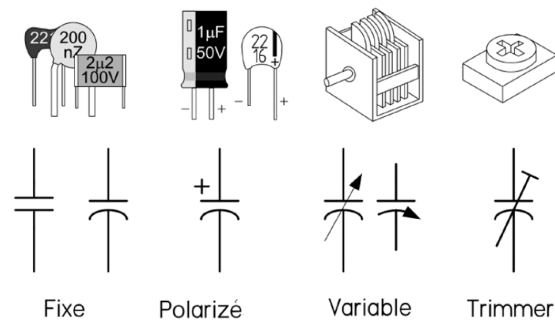
FIGURE 2.4 – Différentes variétés de condensateurs.
