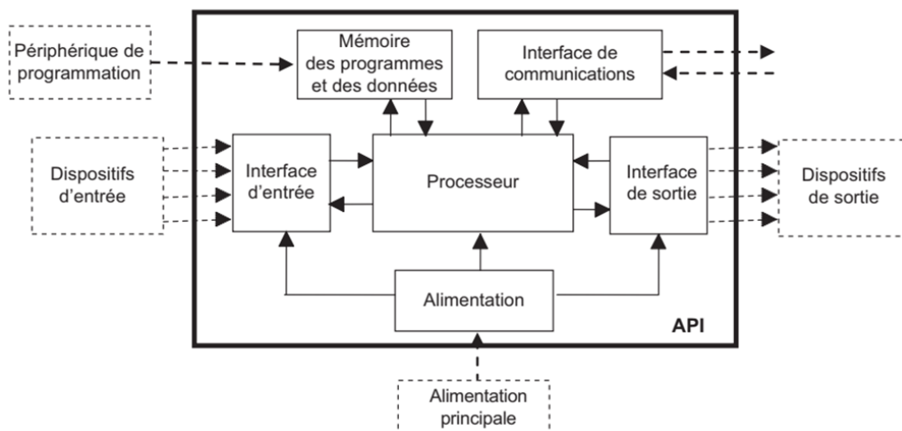
FIGURE 5.5 – Structure d'un API [24].
