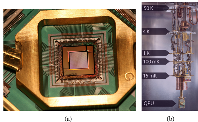
FIGURE 2.14 – Ordinateur quantique D-Wave-2000Q : (a) QPU (Quantum Processing Unit) et (b) ordinateur quantique D-Wave-2000Q, où à partir de la température ambiante en haut (en Kelvin), la température diminue à chaque niveau jusqu'à ce qu'elle soit proche du zéro absolu au niveau du QPU .[3]
