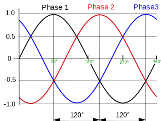
FIGURE 4.1 – Système triphasé équilibré : lorsque les trois conducteurs sont parcourus par des courants de même valeur efficace, le système est dit équilibré. ©Contenu soumis à la licence CC-BY-SA 3.0. Source : Article Réseau électrique de Wikipédia en français.
